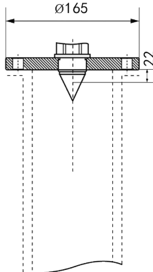
DN150
