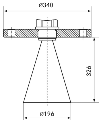
DN200
